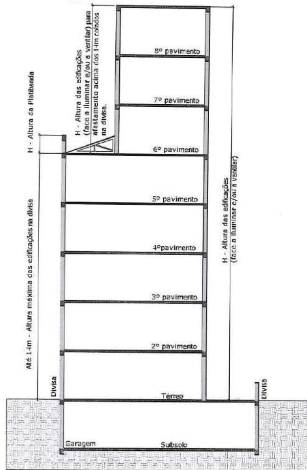
Figura 23A - O diâmetro mínimo para afastamento da face a ventilar e/ou iluminar acima dos 14 m (quatorze metros).
