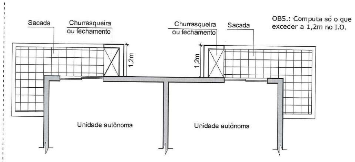
Figura 14 – Sacadas.
