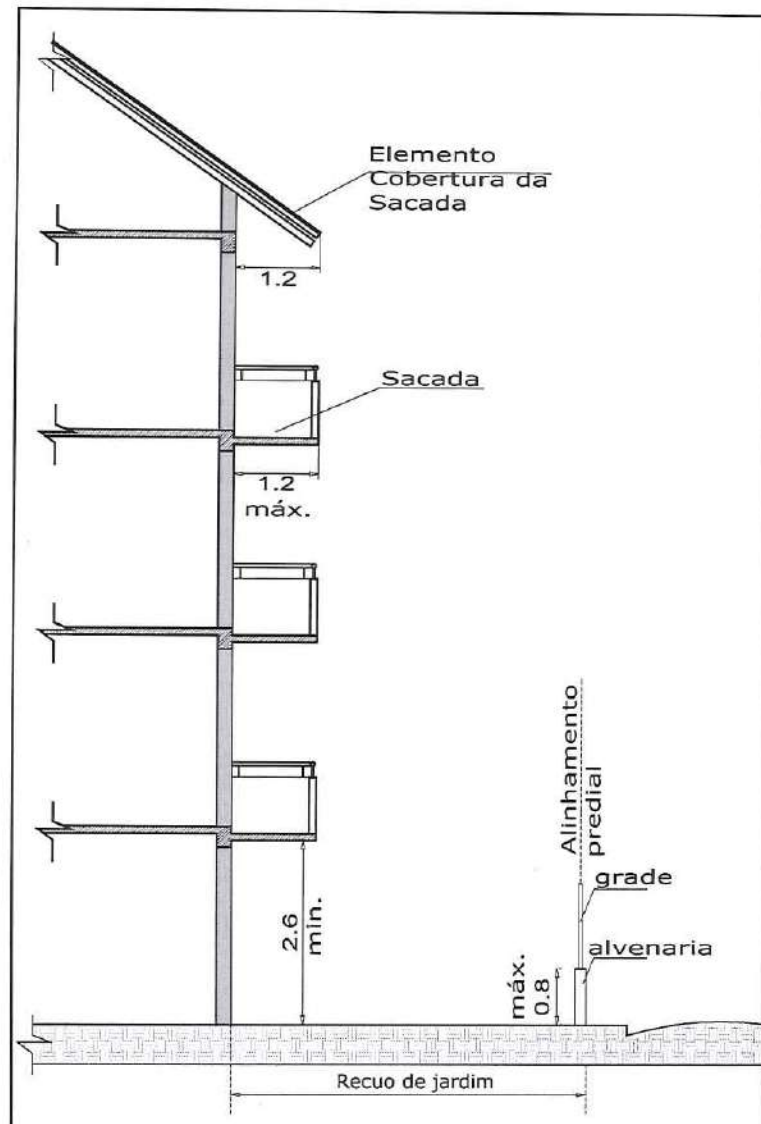
Figura 9 – Sacadas e beirais. 8
