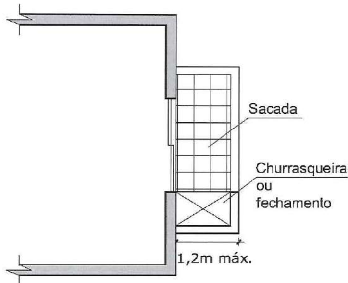
Figura 10 – Sacada.
