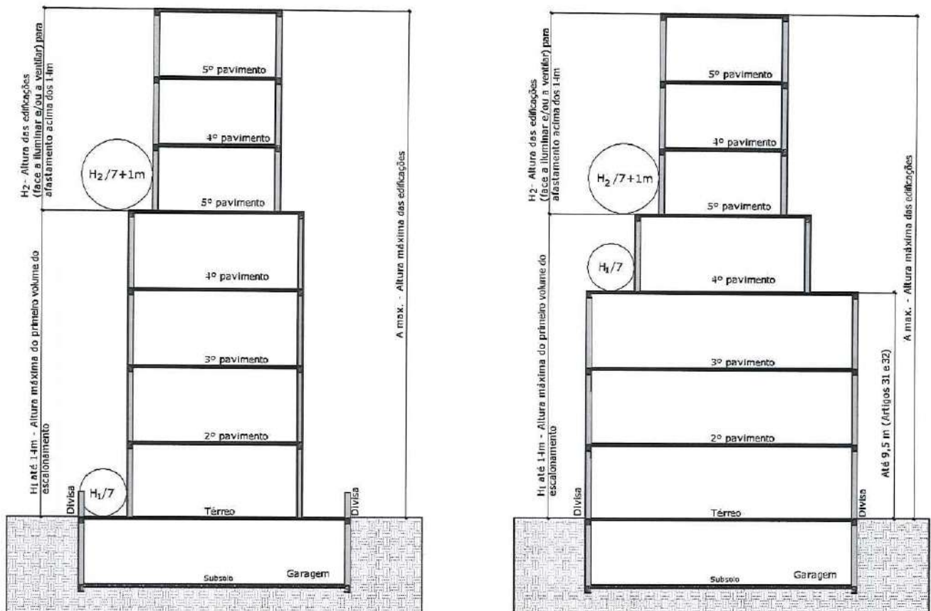
Figura 21A - Afastamento em edificações escalonadas.
