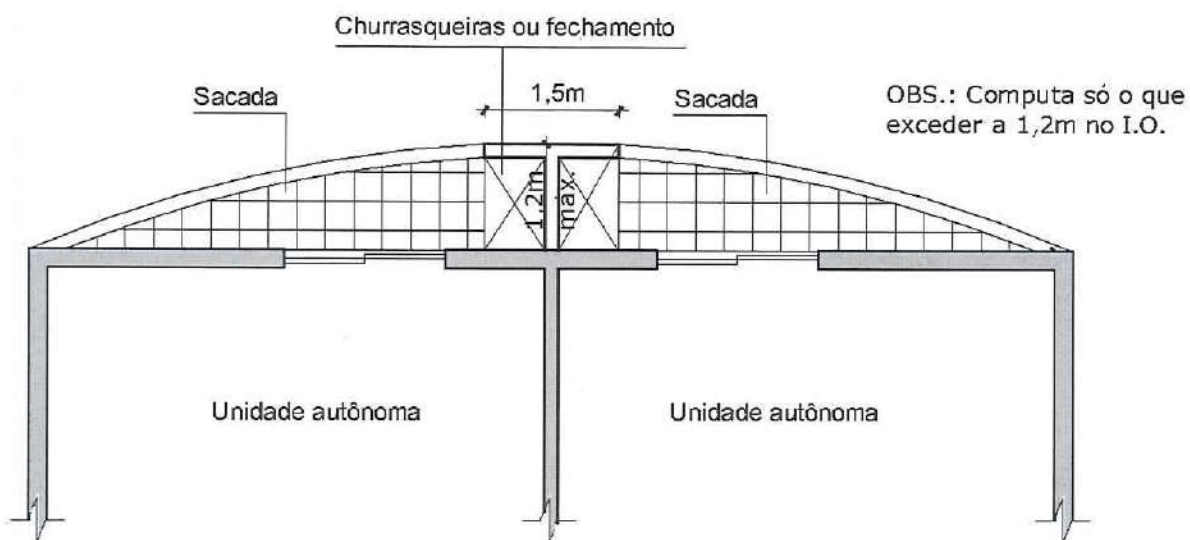
Figura 13 – Sacadas.
